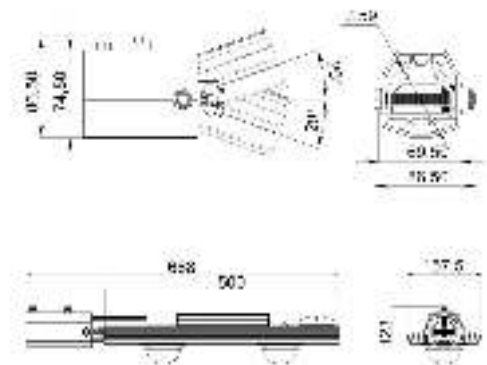
Габаритный чертеж
