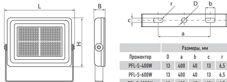
Рис. 1. Прожектор PFL-S
