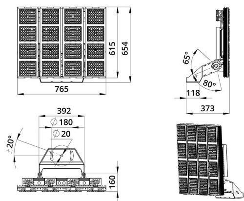
Габаритный чертеж
