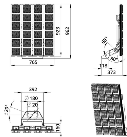
Габаритный чертеж
