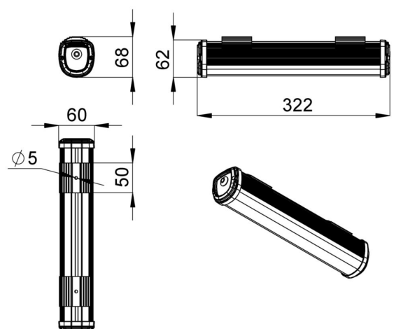
Габаритный чертеж
