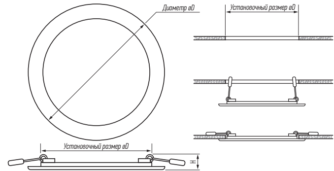
Рис. 1. Светильник PPL-R
